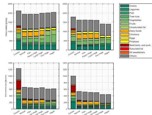
図 男女別・食習慣別の最適化計算の結果。 上は日平均食品摂取量、下は CF。
